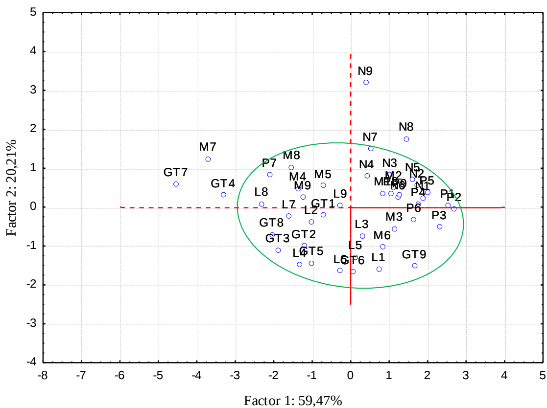
Slika 16. Grafički prikaz odnosa faktora 1 (PCA1) i faktora 2 (PCA2) za ispitivane biljne ekstrakte s obzirom na udjel određivanih bioaktivnih parametara kao pokazatelja ekstrakcijske učinkovitosti
