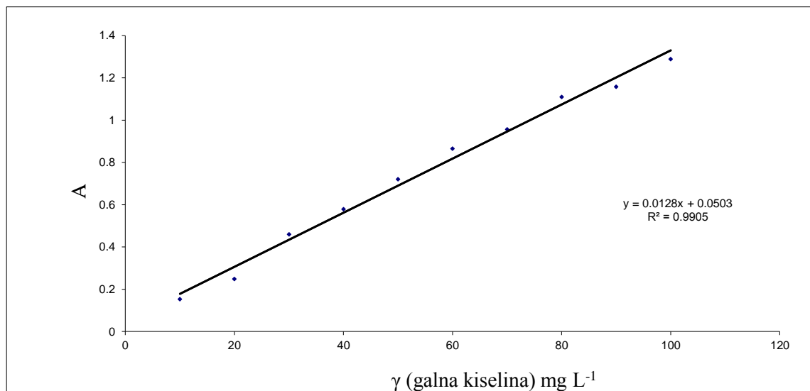
Slika 9. Baždarni dijagram za galnu kiselinu s pripadajućim baždarnim pravcem koeficijentom determinacije ( R^2 )
