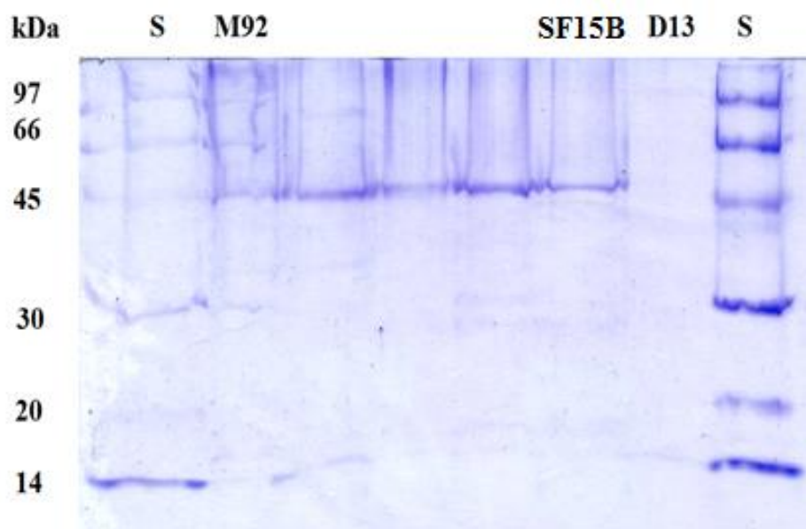
Slika 21. Ispitivanje prisutnosti SLAP proteina provođenjem SDS-PAGE elektroforeze nakon druge dijalize; S-standard; M92- L. helveticus ; SF15B – L. brevis ; D13 – L. plantarum .
