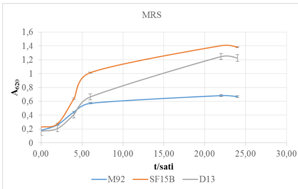
Slika 8. Rast probiotičkih sojeva Lactobacillus helveticus M92, Lactobacillus brevis SF15B i Lactobacillus plantarum D13 u čisto MRS tekućoj podlozi.
