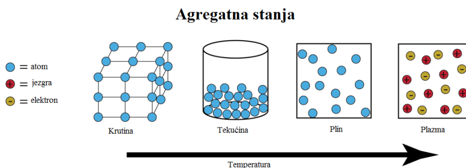
Slika 1. Plazma - četvrto agregatno stanje (Anonymous, 2016b)
