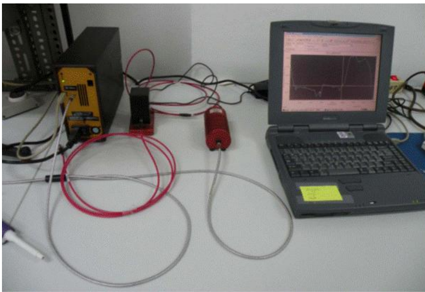
Slika 4. Oprema korištena za snimanje NIR spektra
