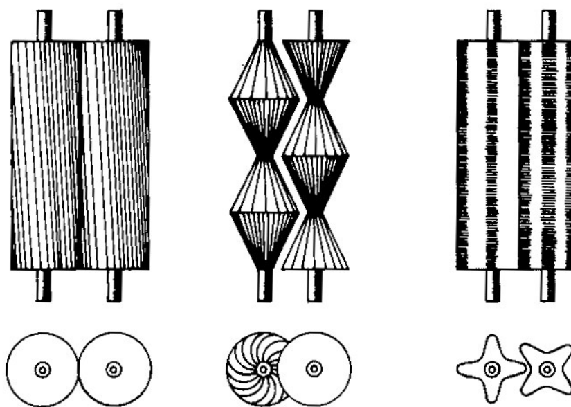
Slika 1. Izgled valjaka raznih tipova muljača (Zoričić, 1996, a).
