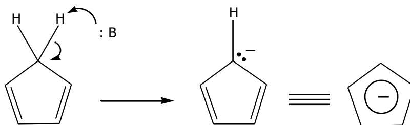
Slika 3. Aromatičnost ciklopentadienilnog prstena ferocena
