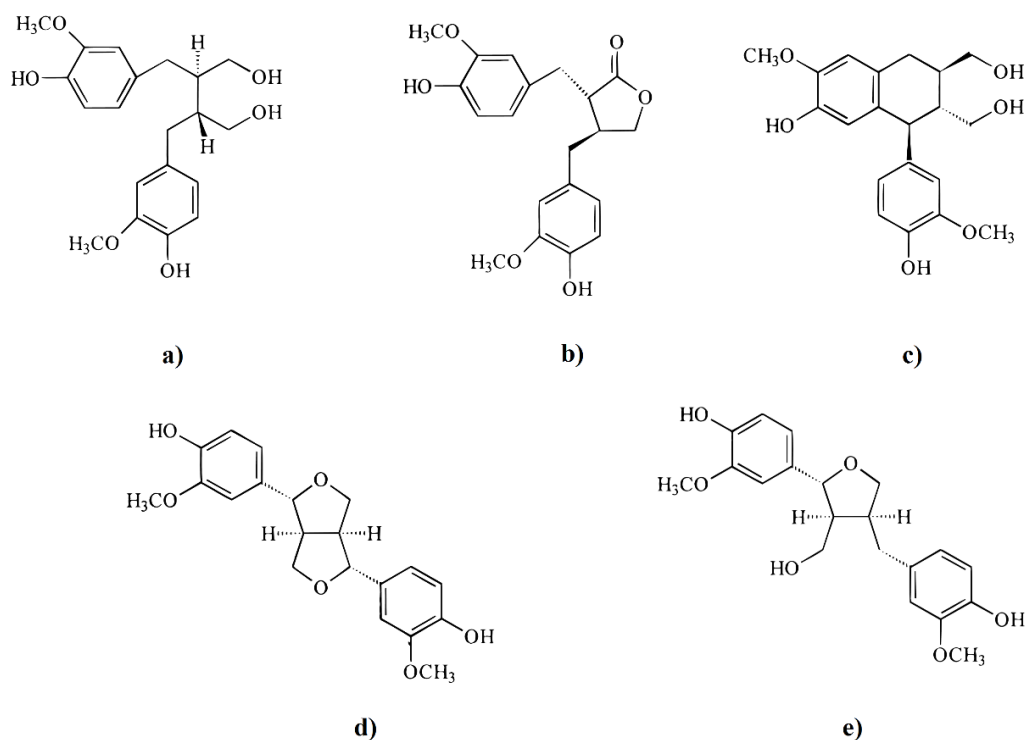
Slika 5. Strukturne formule lignana: a) sekoizolaricirezinol, b) matairezinol, c) izolaricirezinol, d) pinosresinol i e) laricirezinol (Meagher i sur., 1999)
