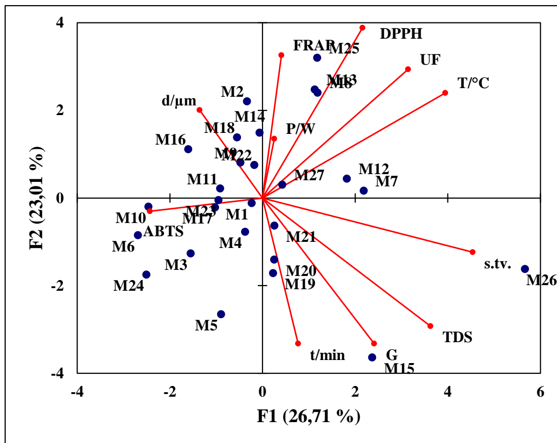
Slika 10. Analiza osnovnih komponenata i promatranih veličina procesa ekstrakcije biološki aktivnih komponenata iz lista masline postupkom ekstrakcije potpomognute mikrovalovima
