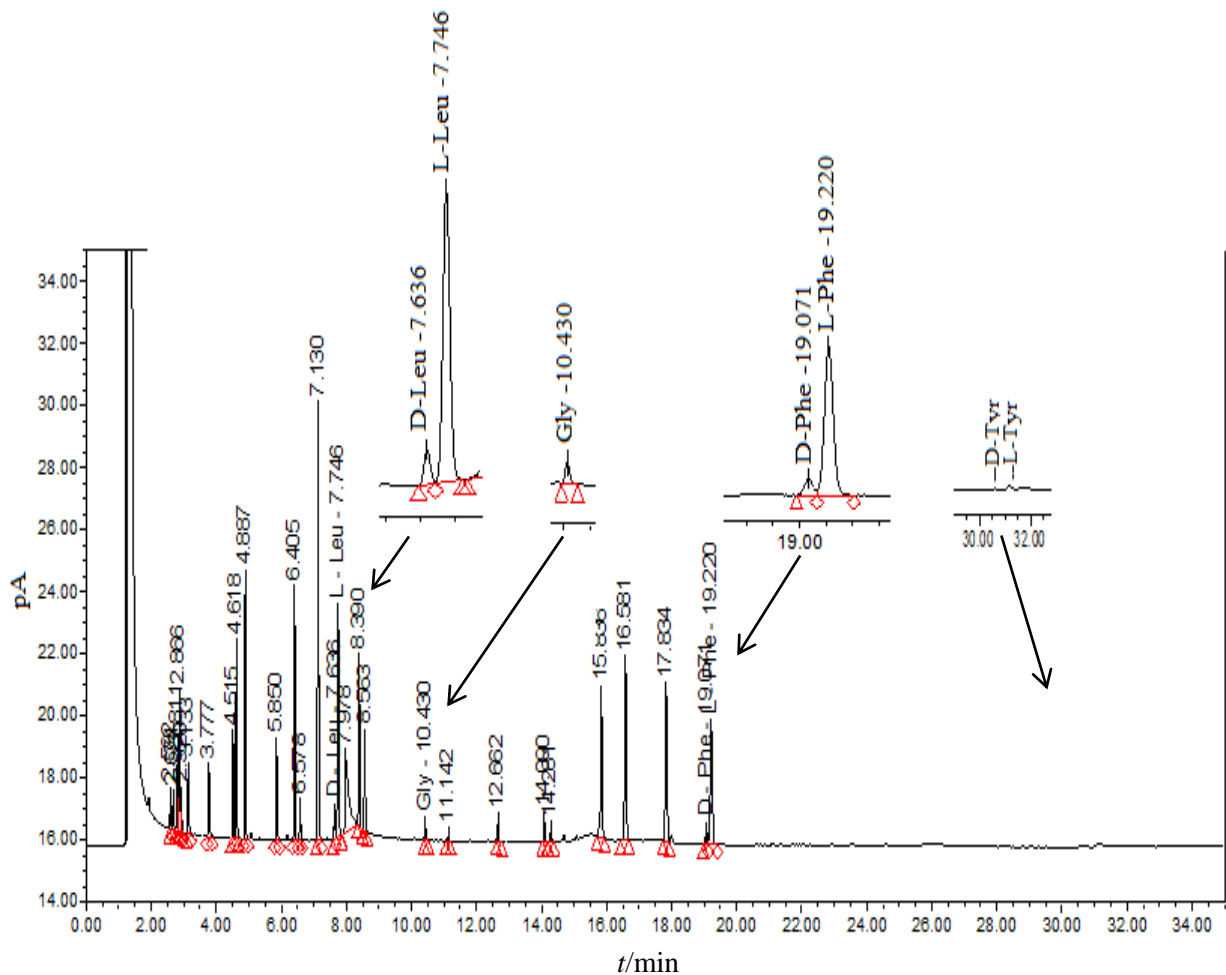
Slika 27. Kromatogram derivata aminokiselina oslobođenih hidrolizom teduglutida na MEGA-DEX DMT beta kromatografskoj koloni, temperaturni program: 80 °C (0 min), povišenje temperature dinamikom od 4 °C/min do 140 °C (20 min).
