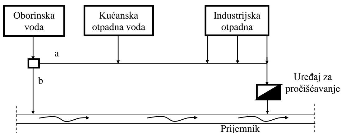
Slika 3. Shematski prikaz polurazdjelnog sustava odvodnje otpadne vode (1)
