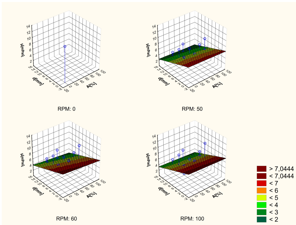
Slika 19. Grafički prikaz utjecaja promjera sonde i amplitude na promjenu viskoznosti (mPas) kategorizirano prema brzini smicanja.
