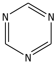
Slika 13. Triazin
