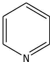
Slika 11. Piridin
