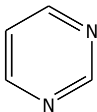
Slika 12. Pirimidin
