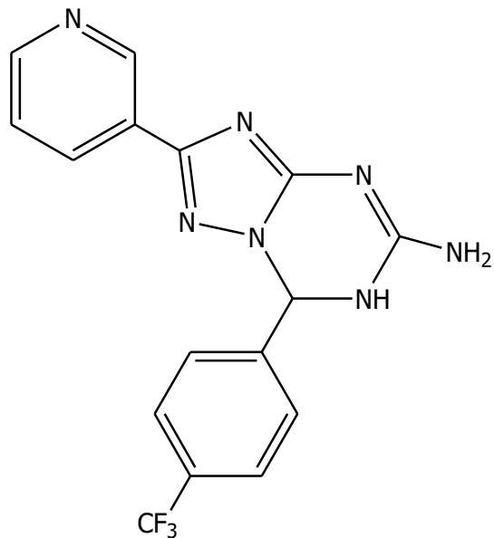
Slika 7. 2-(piridin-3-il)-7-(4-triflorometilfenil)6,7-dihidro[1,2,4]triazolo[1,5-alfa][1,3,5]triazin-5-amin
