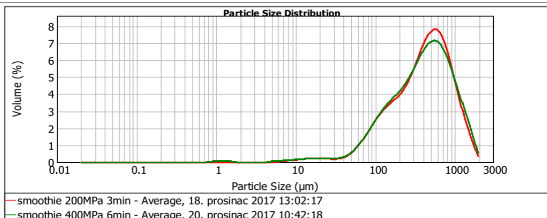
Slika 18. rezultati raspodjele veličina čestica – smoothie 200 MPa/3 min i 400 MPa/6 min
