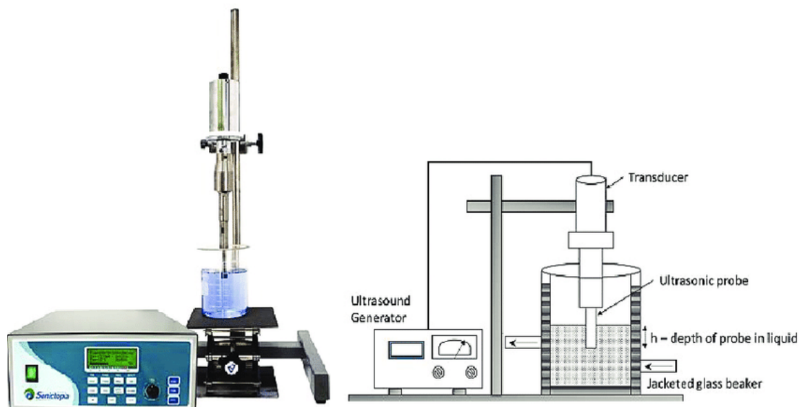
Slika 5. Shematski prikaz i oprema ultrazvučno potpomognute ekstrakcije (Molina i sur., 2016)
