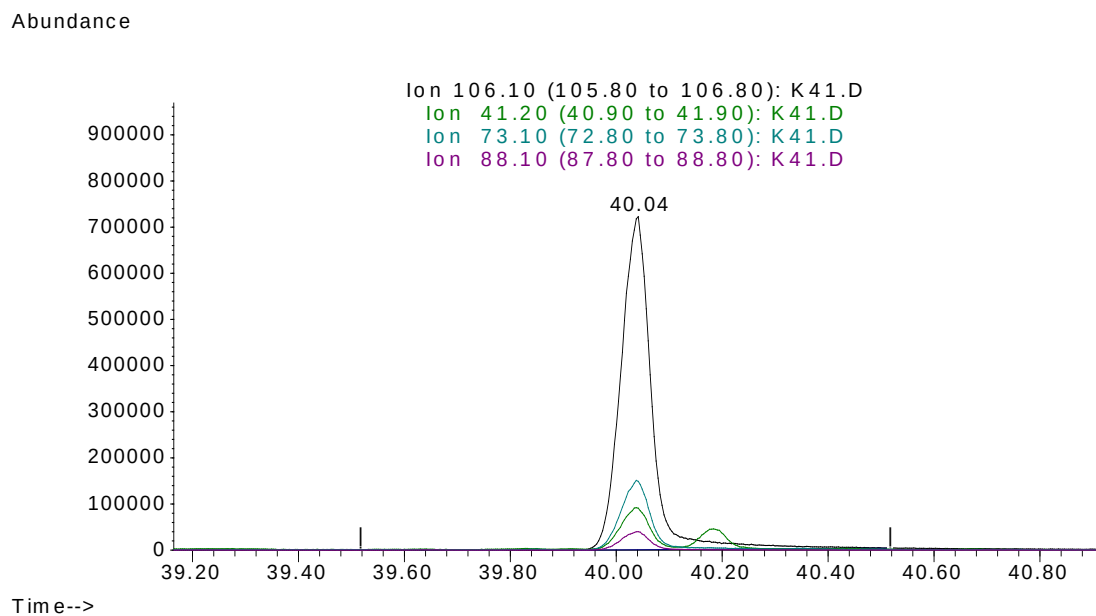
Slika 49. Prikaz kromatograma ciljanog i kvalifikacijskih iona za 3-metiltio-1-propanol
