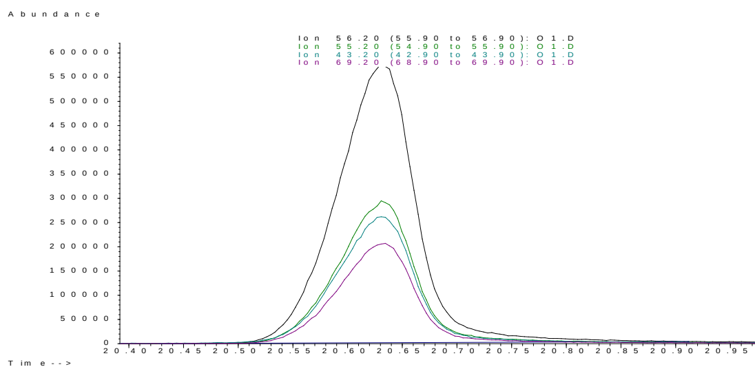
Slika 46. Prikaz kromatograma ciljanog i kvalifikacijskih iona za 1-heksanol
