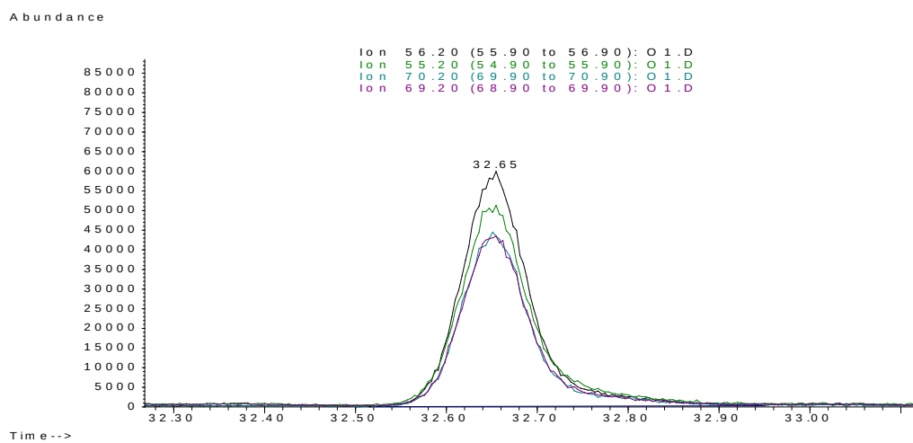
Slika 34. Prikaz kromatograma ciljanog i kvalifikacijskih iona za 1-oktanol
