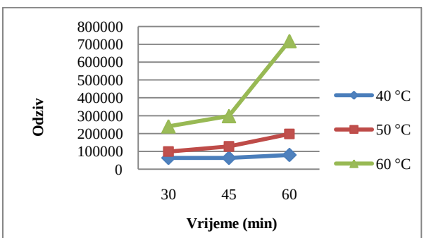
Slika 23. Grafički prikazi ovisnosti odziva 2-nonen-1-ola, cis o vremenu trajanja i temperaturi mikroekstrakcije
