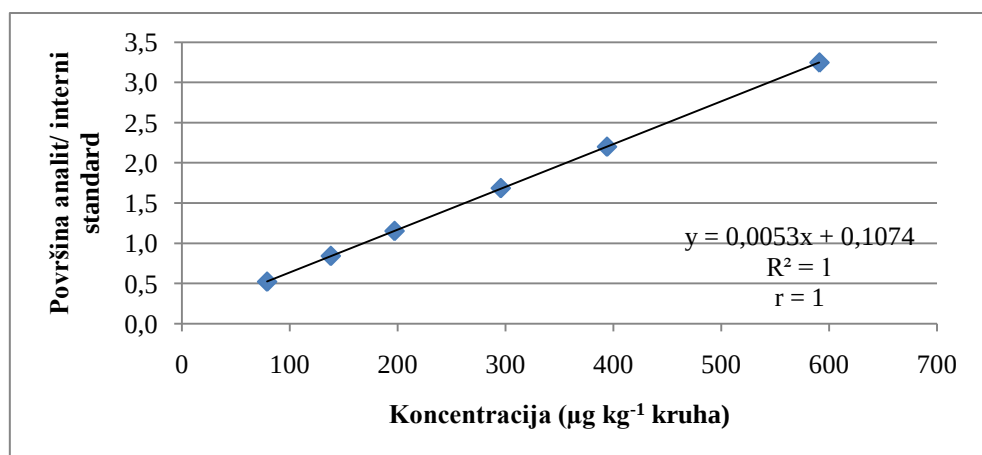
Slika 68. Ovisnost omjera površine i internog standarda o koncentraciji 1-pentanol
