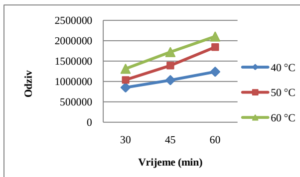
Slika 19. Grafički prikazi ovisnosti odziva 2-metil pirazina o vremenu trajanja i temperaturi mikroekstrakcije
