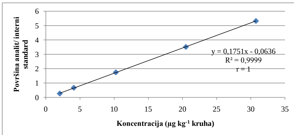
Slika 59. Ovisnost omjera površine i internog standarda o koncentraciji 2-okten-1-ol, transa
