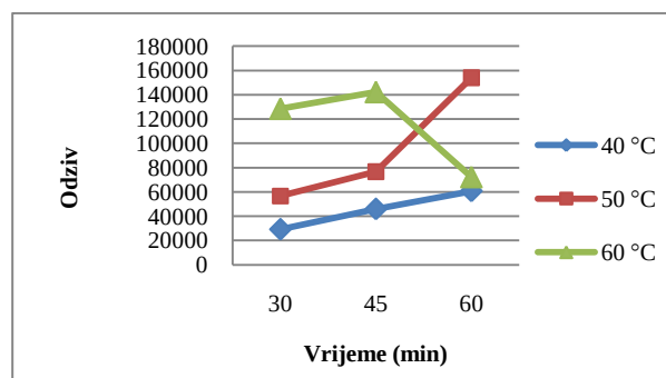
Slika 22. Grafički prikazi ovisnosti odziva 3-metiltio-1-propanola o vremenu trajanja i temperaturi mikroekstrakcije
