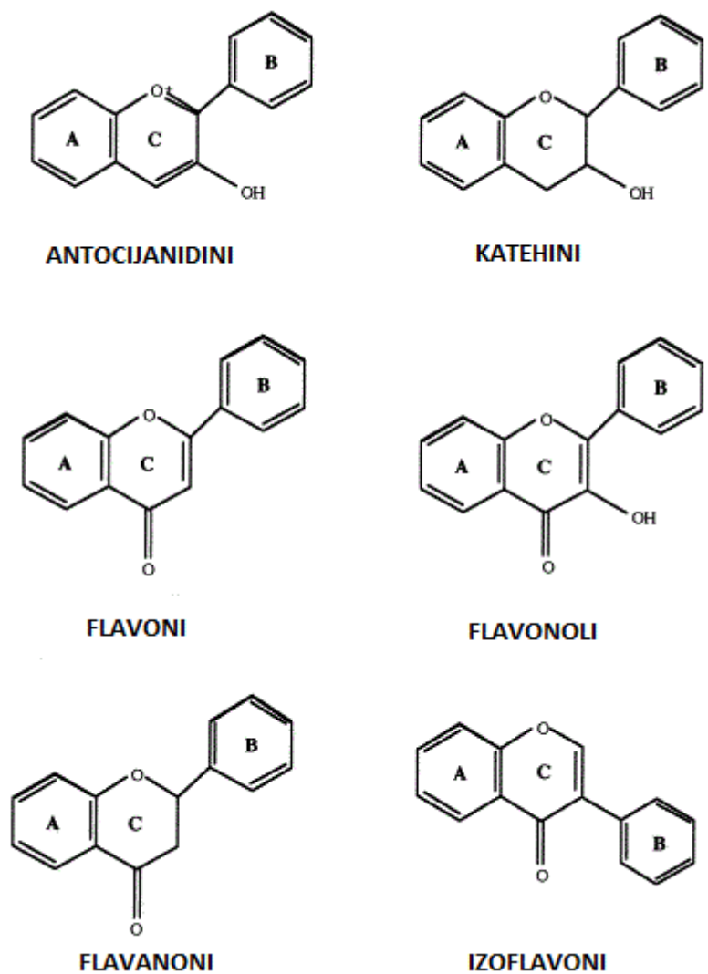
Slika 3. Klasifikacija flavonoida s obzirom na varijacije u heterocikličkom prstenu C (prema Aisling Aherne i O'Brien, 2002)
