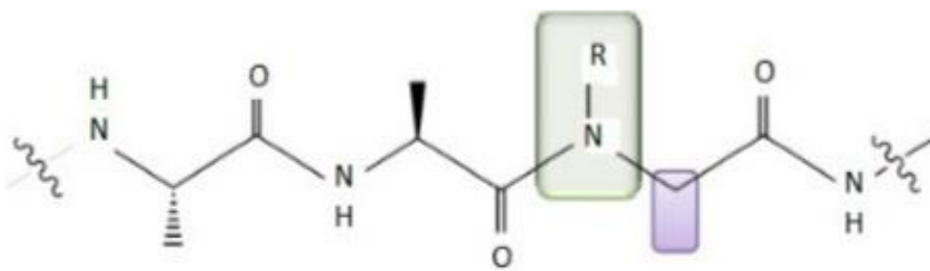
Slika 1. Peptoid
