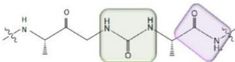
Slika 2. Ureidopeptid
