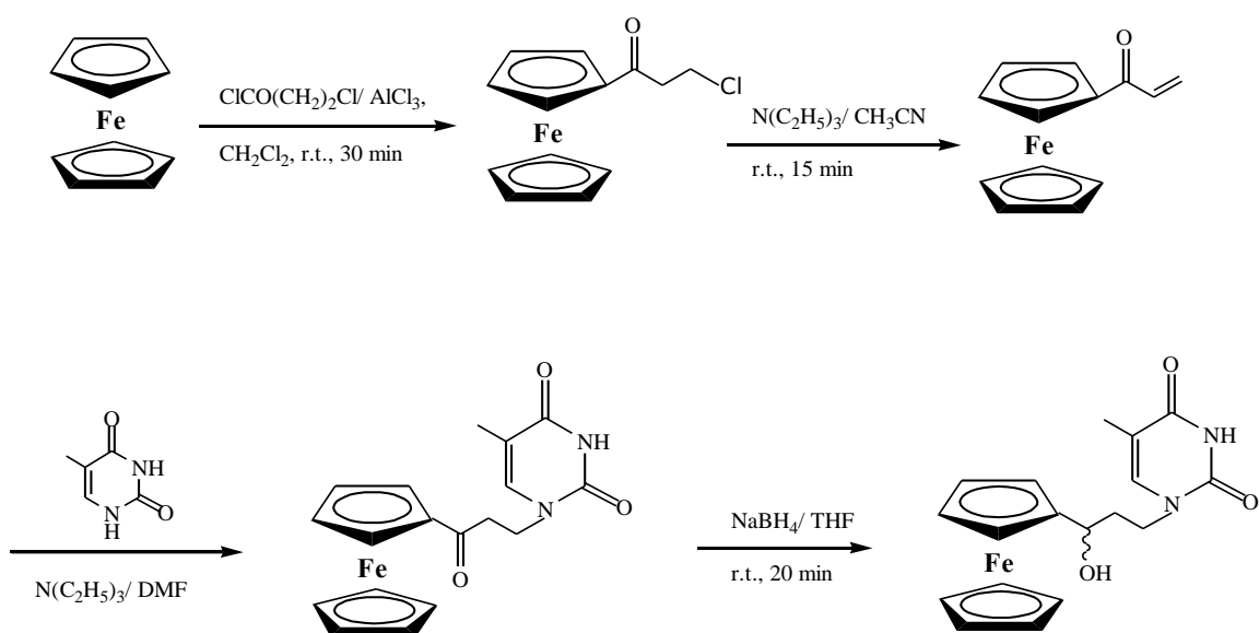
Slika 11. Shema reakcije Michaelove adicije akriloferoceca s timinskom nukleobazom [34]
