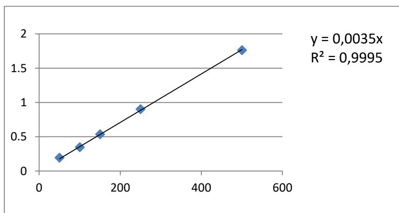
Slika 8. Baždarni pravac za određivanje ukupnih fenola
