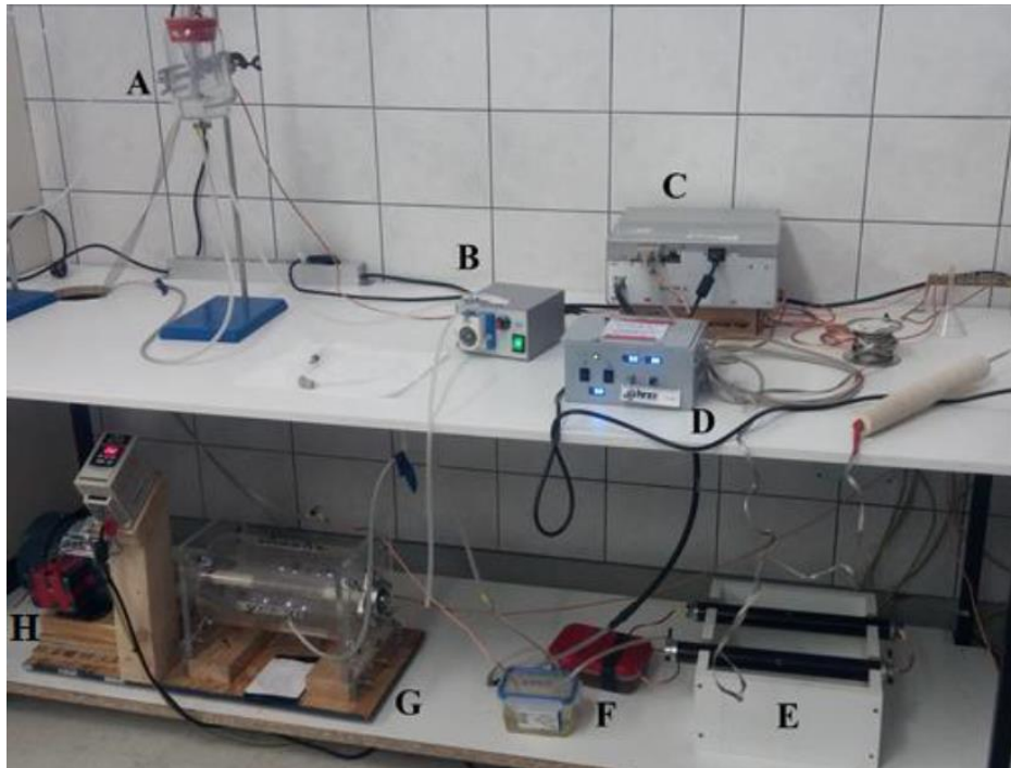
Slika 6. Sustav za generiranje plazme u tekućini visokonaponskim pražnjenjem: A) reaktor, B) pumpa, C) visokonaponski generator, D) kontrolna jedinica za napajanje, E) otpornici 9,5\text{ M}\Omega , F) kondenzator 0,75\text{ nF} , G) rotirajuća sklopka, H) elektromotor s regulatorom frekvencije (arhiva Laboratorija za procesno-prehrambeno inženjerstvo).
