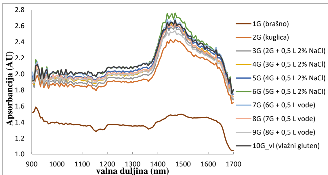
Slika 7. NIR spektri uzoraka nastalih u procesu određivanja vlažnog glutena u glatkom pšeničnom brašnu
