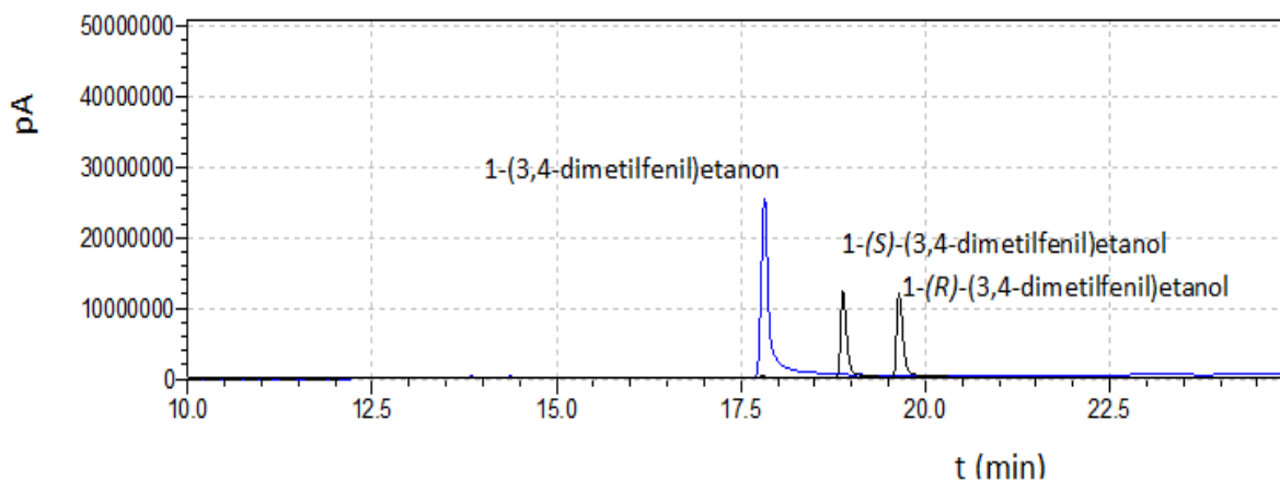
Slika 10. Tipičan GC kromatogram analize reakcijske smjese enantioselectivne redukcije 1-(3,4-dimetilfenil)etanona
