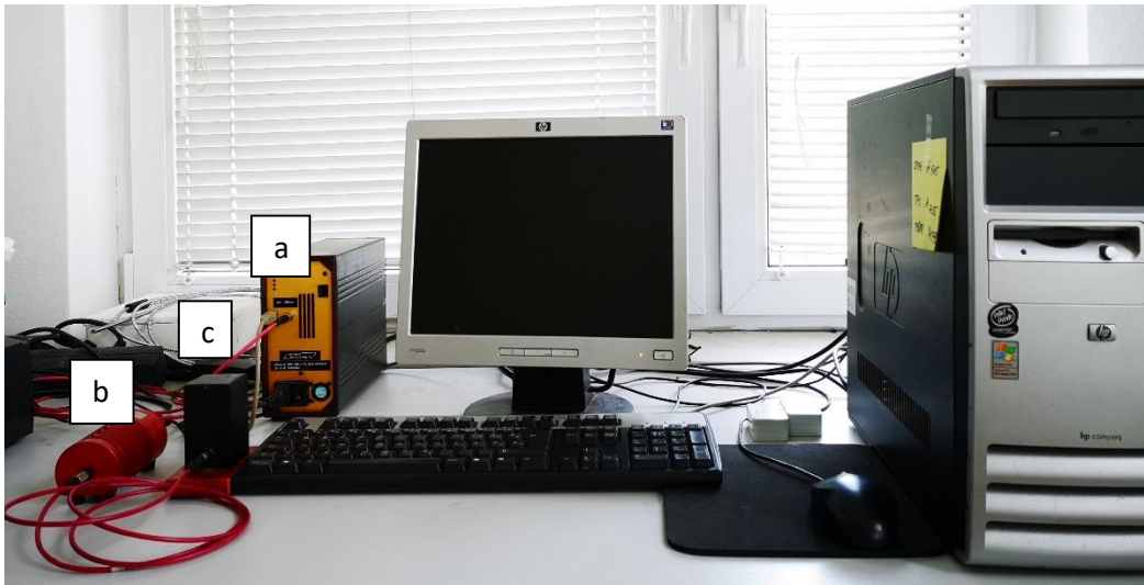
Slika 5. Vlastita fotografija NIR instrumenta spojenog na računalu sa instaliranim programom SPEC-32 (a), izvor zračenja (b) i kućište s kivetom (c)
