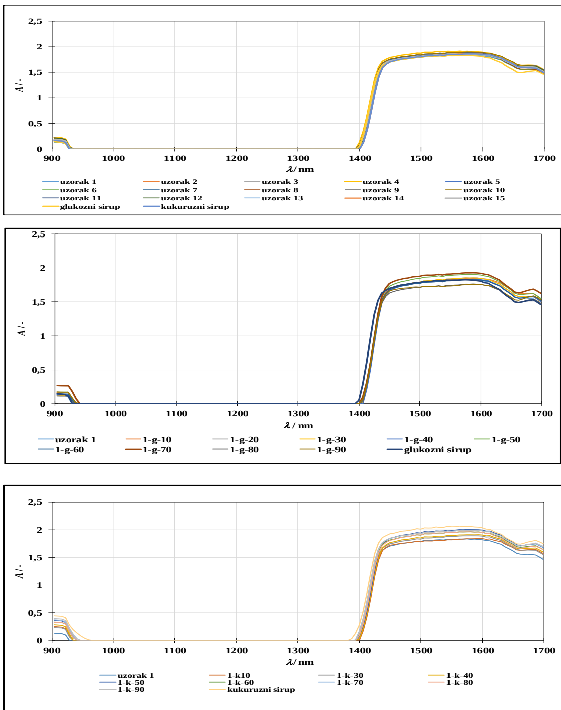
Slika 9. NIR spektri (a) analiziranih uzoraka meda te glukoznog i kukuruznog sirupa, (b) pripremljenih patvorina meda iz uzorka 1. - patvorine s glukoznim sirupom, (c) pripremljenih patvorina meda iz uzorka 1. - patvorine s kukuruznim sirupom
