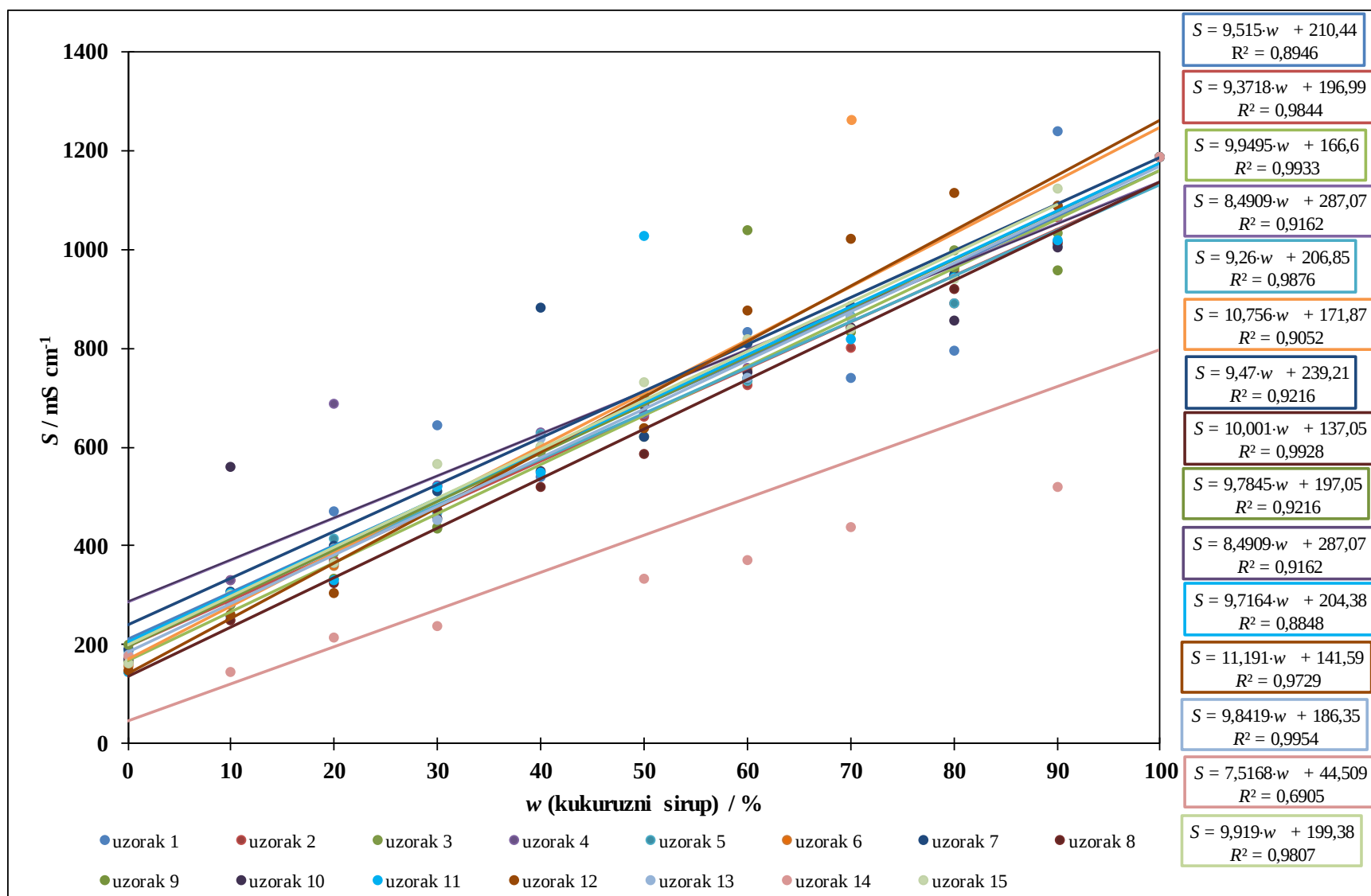
Slika 8. Linearna zavisnost udjela dodanog kukuruznog sirupa i vodljivosti patvorenog meda
