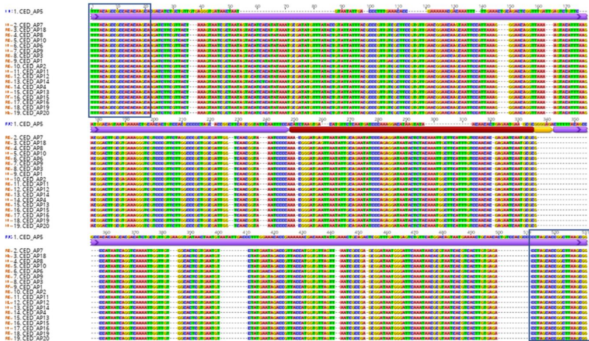
Slika 13. Svrstavanje sekvenci DNA nesrodnih TRIM elementu detektiranih kod vrste C. edule . Prikazani su u odnosu na TRIM element porijeklom iz CED_AP5 klon. TDR domene TRIM elementa su označene ljubičastom, unutarnja domena crvenom, a polipurinski trakt žutom bojom. Vidljiva je visoka homologija između dva tipa sekvenci na njihovim krajevima (obilježeno plavim kvadratima).
