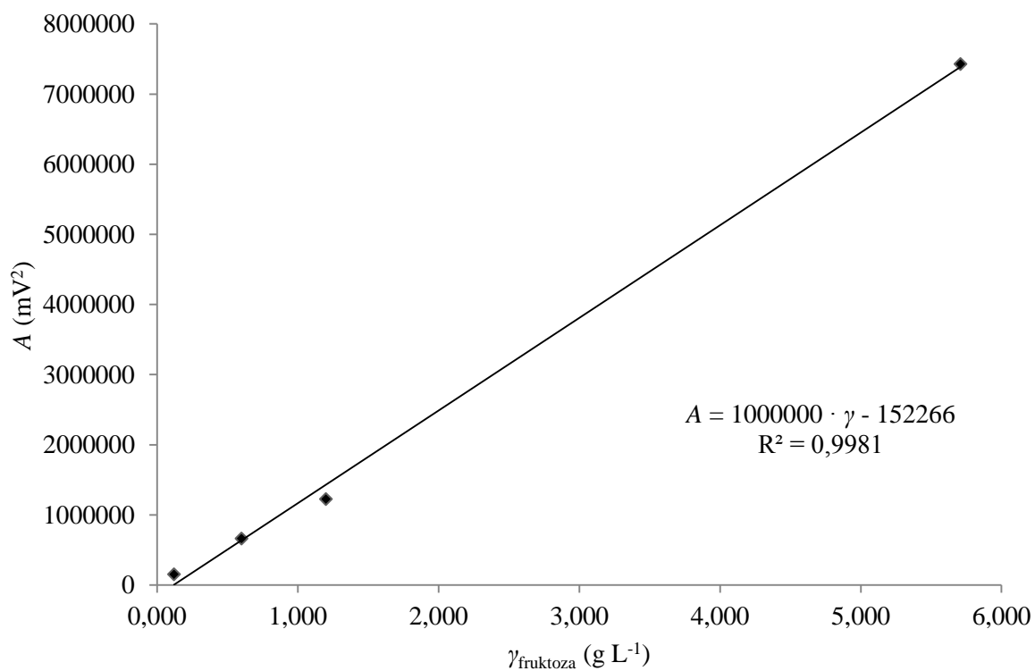
Slika 34. Baždarni dijagram ovisnosti površine pika ( A , \text{mV}^2 ) fruktoze ( t_R = 5,69 min) o njenoj koncentraciji ( \gamma_{\text{fruktoza}} , \text{g L}^{-1} ) u otopini.
