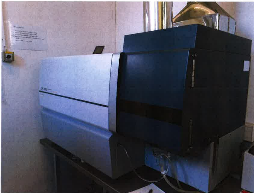
Slika 8. ICP-OES
