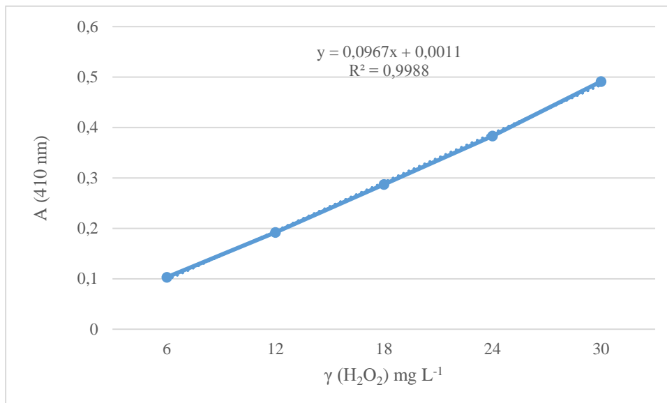
Slika 13. Baždarni dijagram za određivanje vodikovog peroksida
