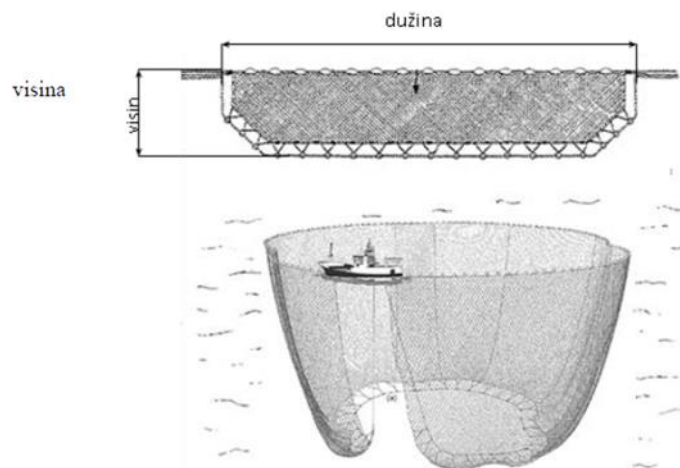
Slika 5. Shematski prikaz okružujuće mreže plivarice (Anonymous, 2014)
