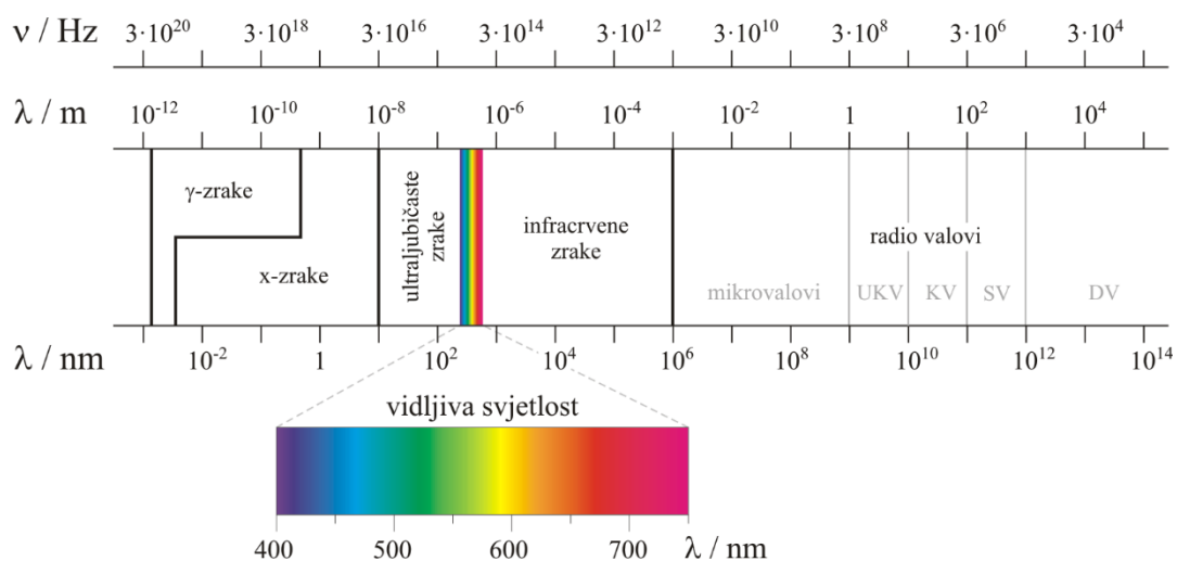
Slika 13. Elektromagnetski spektar zračenja (Anonymous 2, 2020)
