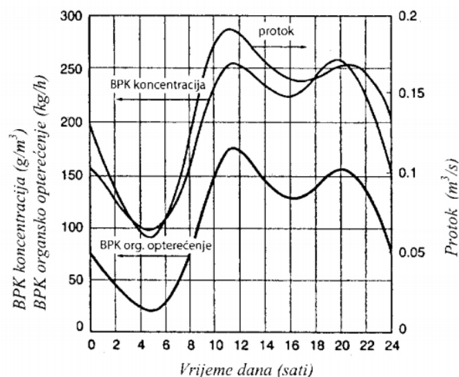
Slika 1. Promjena količine otpadne vode i onečišćenja gdje je BPK 5 izražen kao koncentracija (g/m 3 ) i kao organsko opterećenje (kg/h) (Tchobanoglous, 1991).
