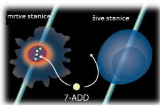
Slika 9. Obilježavanje zdravih i apoptotičnih stanica primjenom Muse® Annexin V & Dead Cell Kit-a: a) vezanje Anenexin V na PS (Anonymous, 2019) i b) ulazak 7-AAD u stanice s oštećenom membranom i mrtve stanice (Anonymous, 2019)
