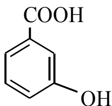
Slika 2. m-hidroksibenzojeva kiselina
