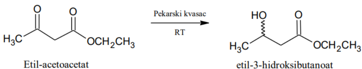
Slika 1. Redukcija etil-acetoacetata u kiralni alkohol etil-3-hidroksibutanoat
