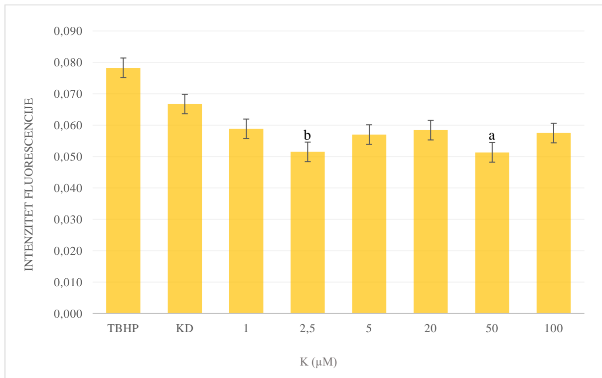
Slika 19. Učinak kurkumina (1-100 µM) na razinu ROS-a u CHO-K1 stanicama 2,5 sata nakon tretmana. Kontrolni uzorci stanica tretirani su tert-butil hidroperoksidom (TBHP) u koncentraciji 50 µM te otapalom dimetil sulfoksidom (DMSO) u koncentraciji 5 µL mL -1 (KD). Podaci su izraženi kao srednja vrijednost ± standardna pogreška. Statistički značajna razlika (Student t -test): a p <0,005, b p <0,025.
