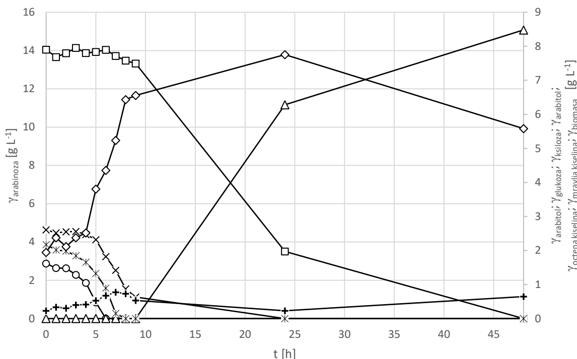
Slika 20. Uzgoj kvasca Spathaspora passalidarum CBS 10155 u bioreaktoru na kiselinskom hidrolizatu izluženih repinih reznaca (—□—arabinoza, —○— glukoza, —×— ksiloza —△— arabitol, —◇— biomasa, —+— mravlja kiselina, —*—octena kiselina, —■— etanol)
