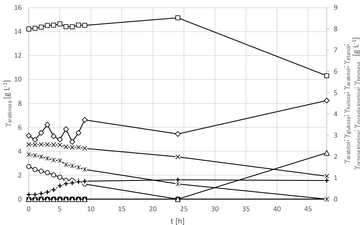
Slika 21. Uzgoj kvasca Spathaspora arborarie CBS 11463 u bioreaktoru na kiselinom hidrolizatu izluženih repinih rezanaca (—□—arabinoza, —○— glukoza, —×— ksiloza —△— arabitol, —◇— biomasa, —+— mravlja kiselina, —*— octena kiselina, —■— etanol)
