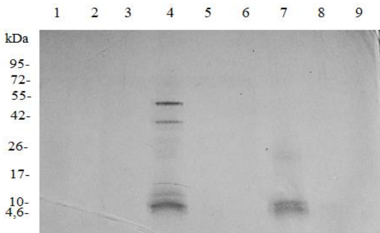
Slika 6. Prikaz gela nakon provedene SDS elektroforeze. Prikazani su uzorci redom: ukupan hidrolizat proteina nakon djelovanja enzima Alcalased (1) te frakcija ispod 10 kDa (2) i ispod 1 kDa(3), ukupan hidrolizat proteina nakon djelovanja enzima Neutrased (4) te frakcija ispod 10 kDa (5) i ispod 1 kDa (6), ukupan hidrolizat proteina nakon djelovanja enzima Protamex (7) te frakcija ispod 10 kDa (8) i ispod 1 kDa (9).
