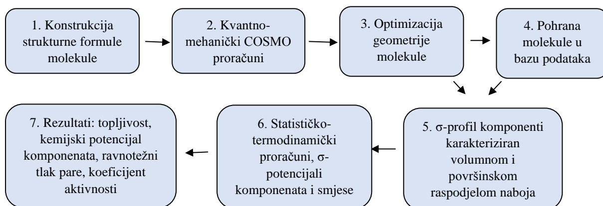
Slika 7. Shematski prikaz dijagrama toka proračuna, unutar programa TMoleX i COSMOtherm
