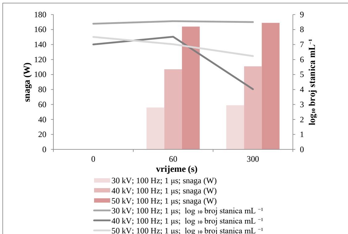
Slika 11. Utjecaj napona, frekvencije (100 Hz), trajanja pulsa (1 \mu s) i snage o vremenu trajanja procesa na inaktivaciju bakterije L. plantarum nakon tretmana pulsirajućim električnim poljem
