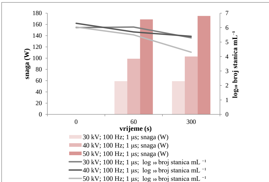
Slika 7. Utjecaj napona, frekvencije (100 Hz), trajanja pulsa (1 \mu s) i snage o vremenu trajanja procesa na inaktivaciju kvasca S.cerevisiae nakon tretmana pulsirajućim električnim poljem
