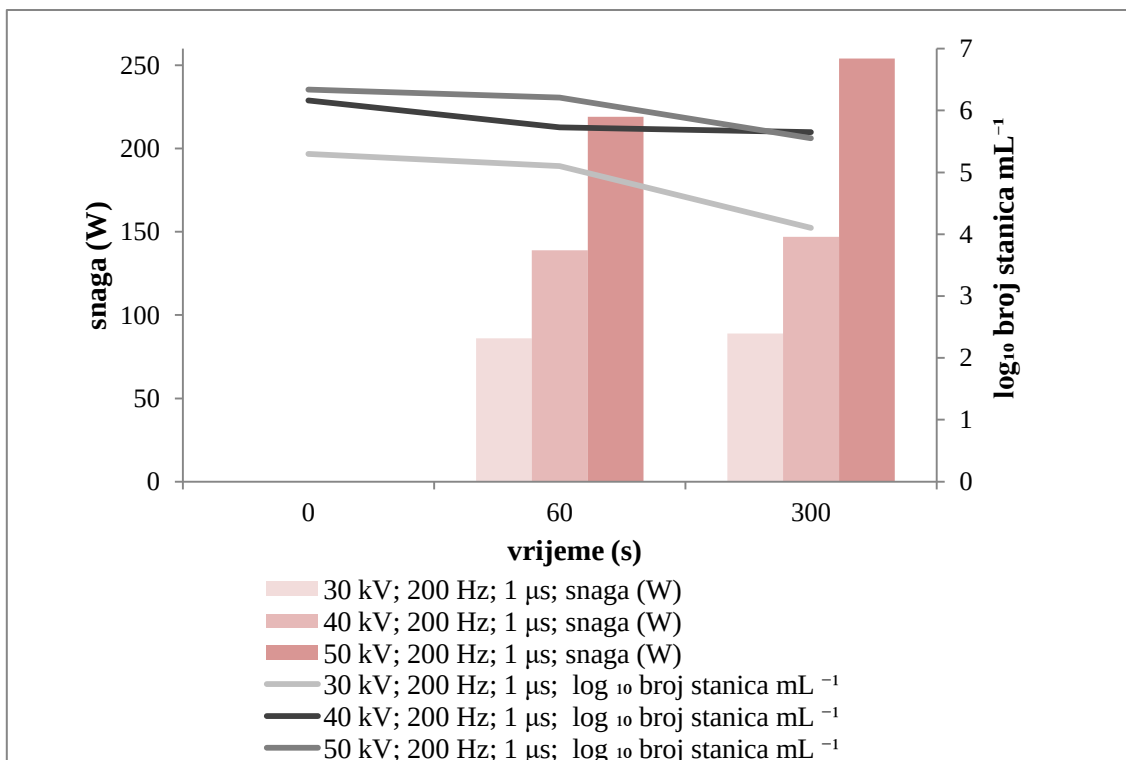
Slika 8. Utjecaj napona, frekvencije (200 Hz), trajanja pulsa (1 \mu\text{s} ) i snage o vremenu trajanja procesa na inaktivaciju kvasca S.cerevisiae nakon tretmana pulsirajućim električnim poljem
