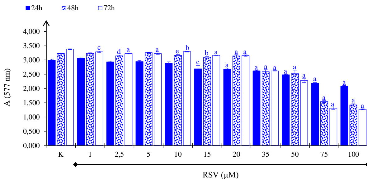
Slika 33. Učinak resveratrola (RSV 1 – 100 μM) na vijabilnost Hepa1-6 stanica 24, 48 i 72 sata nakon tretmana određen metodom Kenacid Blue . Rezultati su prikazani kao srednja vrijednost apsorbancije pri 577 nm ± standardna pogreška (K – stanice tretirane s 5 μL DMSO-a mL -1 medija za uzgoj; 1 – 100 – stanice tretirane resveratrolom u koncentracijama od 1 – 100 μM). Statistički značajna razlika u odnosu na K (Student t -test): e p<0,05, d p<0,025, c p<0,01, b p<0,005, a p<0,001.
