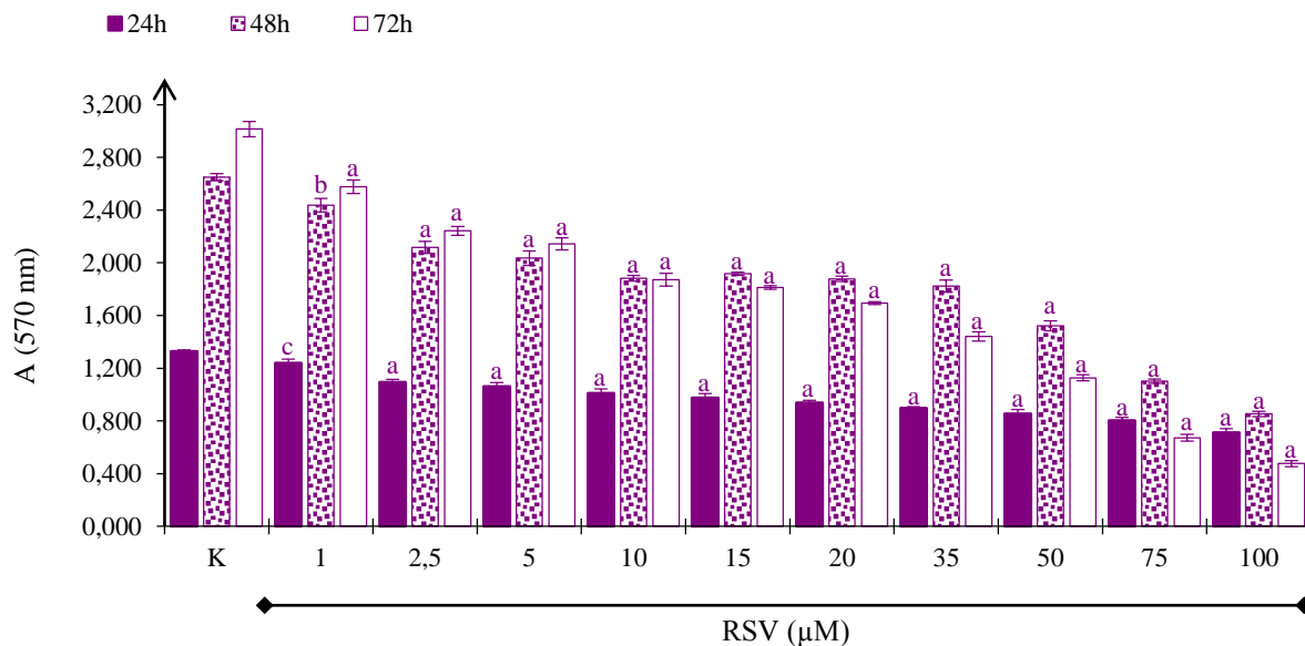
Slika 34. Učinak resveratrola (RSV1 – 100 μM) na vijabilnost Hepa1-6 stanica 24, 48 i 72 sata nakon tretmana određen metodom MTT . Rezultati su prikazani kao srednja vrijednost apsorbancije pri 570 nm ± standardna pogreška (K – stanice tretirane s 5 μL DMSO-a mL -1 medija za uzgoj; 1 – 100 – stanice tretirane resveratrolom u koncentracijama od 1 – 100 μM). Statistički značajna razlika u odnosu na K (Student t -test): c p<0,025, b p<0,005, a p<0,001.
