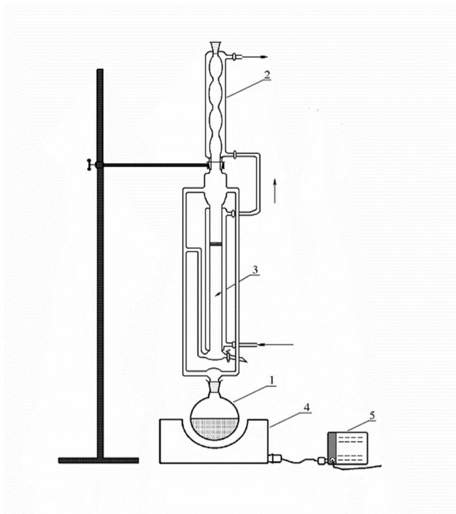
Slika 12. Modificirana aparatura po Clevengeru za hidrodestilaciju (1. tikvica s okruglim dnom; 2. povratno hladilo; 3. prostor za prihvat destilata; 4. kalota za zagrijavanje, 5. reostat) (Zekić, 2013).
