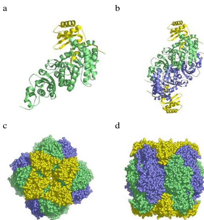
Slika 1. Raspored podjedinica heksadekamskog proteina RuBisCO-a. L podjedinice prikazane su zelenom i plavom bojom, a S podjedinice žutom. (a) Jedna L i jedna S podjedinica. (b) Dvije jedinice LS kompleksa. (c) Prikaz potpunog holoenzima (L8S8). (d) Prikaz holoenzima okomitog u odnosu na prikaz pod (c). (preuzeto i prilagođeno iz Karkehabadi, 2005)
