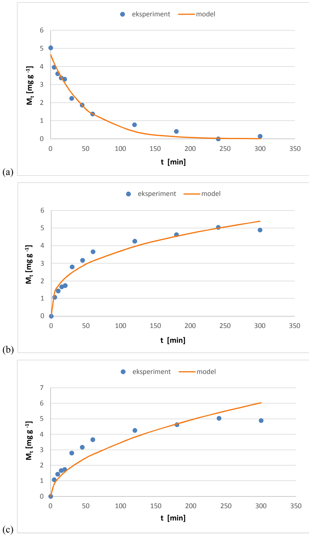
Slika 20. Kinetički modeli desorpcije BSA: (a) prvi red, (b) Korsmeyer-Peppas i (c) Higuchi
