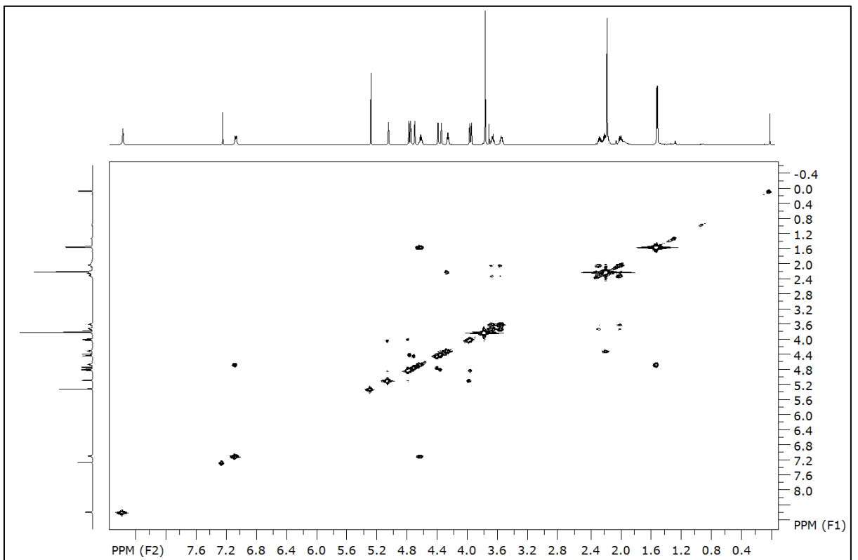
Slika 8. 1 H- 1 H COSY NMR-spektar peptida 4 ( c = 5 \times 10^{-2} M).
