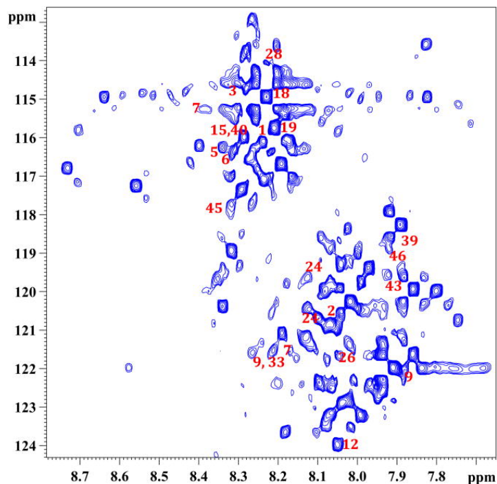
Slika 7. Dio spektra ^1\text{H} - ^{15}\text{N} HSQC ljudskog urina označenog sa ^{15}\text{N} -kolaminom. 1: akonitinska kiselina; 2: adipinska kiselina; 3: alanin; 5: arginin; 6: asparagin; 7: asparaginska kiselina; 9: limunska kiselina; 12: mravlja kiselina; 15: glutaminska kiselina; 18: glikolna kiselina; 19:
