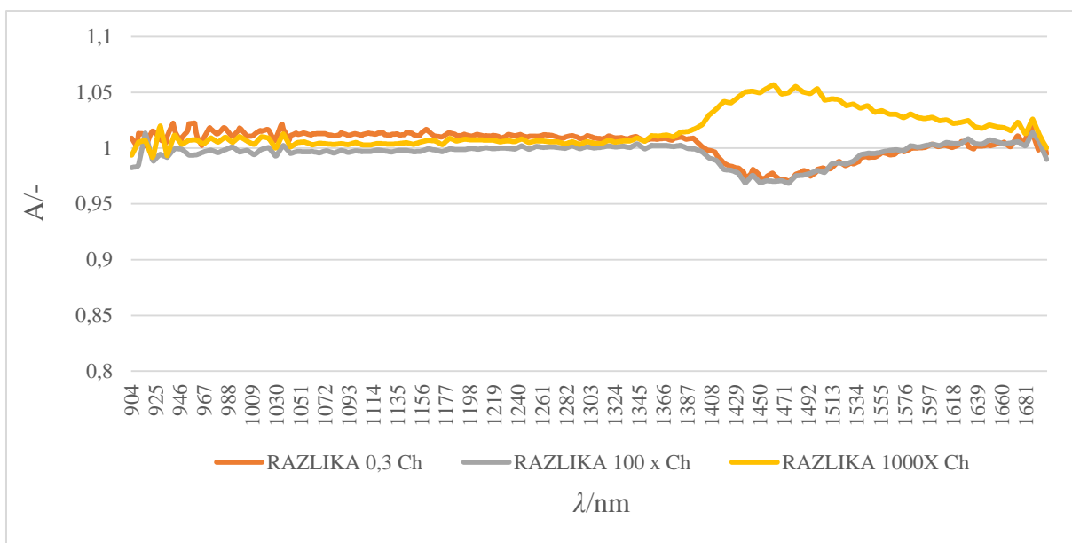
Slika 23. Prikaz NIR spektara kontaminiranih jabuka (Chromosul 80) nakon što su se srednje vrijednosti njihovih apsorbancija umanjile za srednje vrijednosti apsorbancija netretiranih jabuka za četrnaesti dan (srednje vrijednosti apsorbancija originalnih suspenzija (RAZLIKA 0,3 Ch) i suspenzija koje su sto (RAZLIKA 100X Ch) i tisuću puta (RAZLIKA 1000X Ch) razrjeđenije od originalne, umanjene za srednje vrijednosti apsorbancija netretiranih jabuka)
