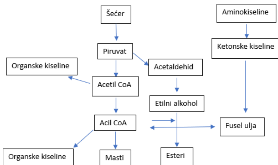
Slika 1. Shematski prikaz nastanka fermentacijskih produkata (prema Tang i Li, 2017)
