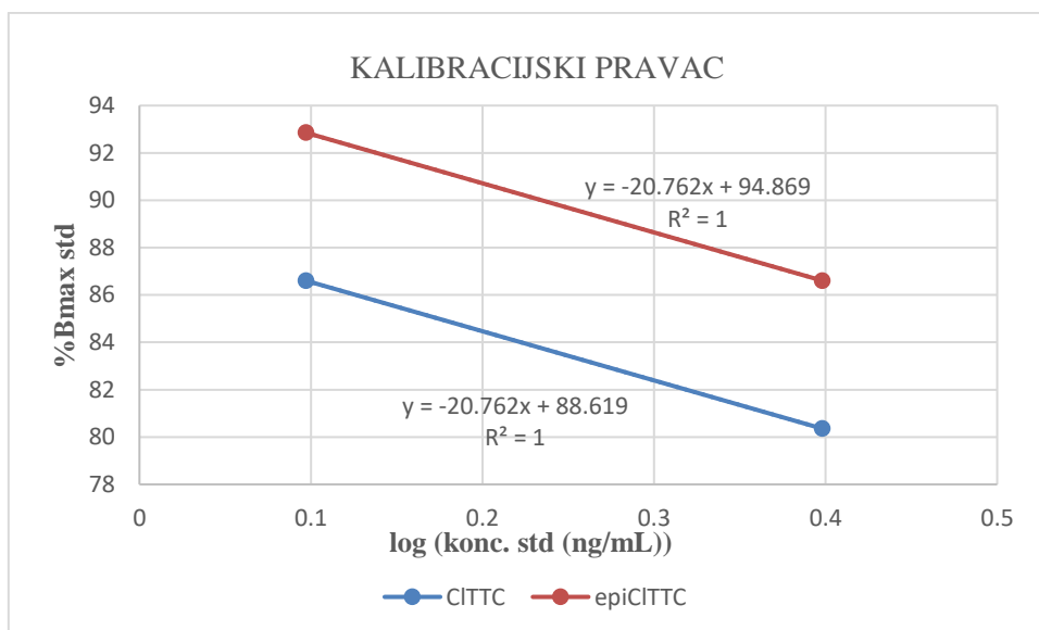
Slika 25. Kalibracijski pravac za standarde klortetraciklina i epiklortetraciklina
