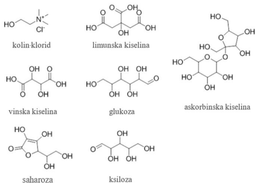
Slika 2. Kemijska struktura različitih spojeva koji se mogu koristiti za pripravu NADES-ova (prema Paiva i sur., 2014)
